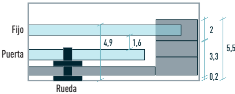
Detalle planta mampara Manhattan
