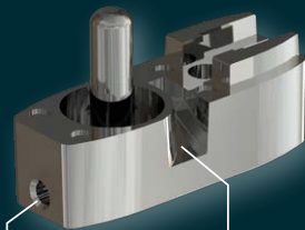
Fijación para alinear la puerta Sistema de desaguo del pivote inferior
