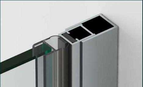
Perfil magnético oculto de compensación incluido
