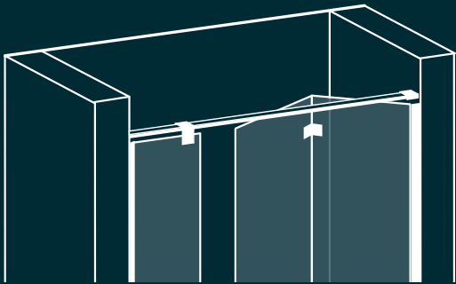
Barra de seguridad de lado a lado para fijo superior a 40 cm.
