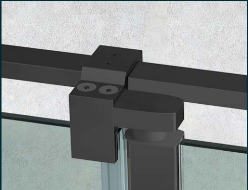
Pinza fijo-pivote superior en Acero Inoxidable 304
