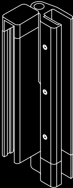
detalle técnico bisagras extended
